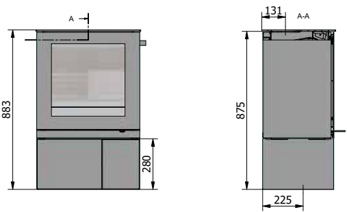
Version avec socle bas
