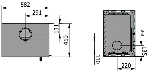
Version avec socle haut
