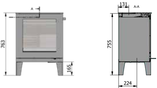
Version avec pieds design haut
